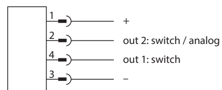
Fig. 18: Wiring diagram
